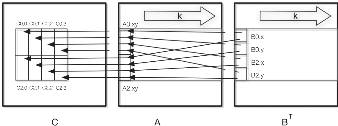
Fig. 8. ATI DGEMM algorithm.
